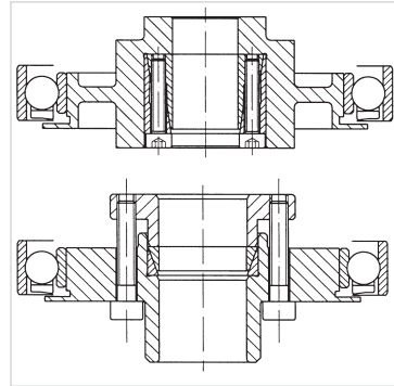
Designbeispiele für Solid Wave Generator mit Spannelement. Design examples for Solid Wave Generator with clamping element.
